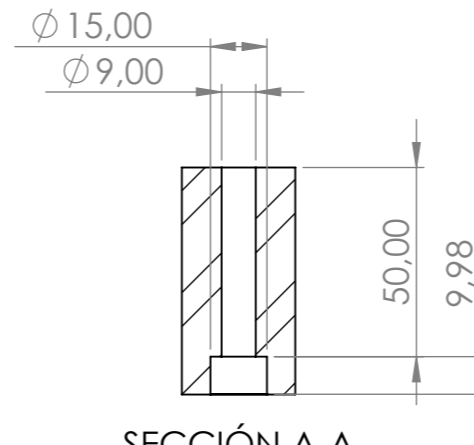
SECCIÓN A-A ESCALA 1 : 2
