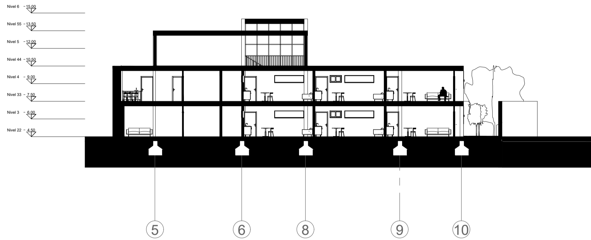
P-09 CORTE CC' ESC. 1:200
