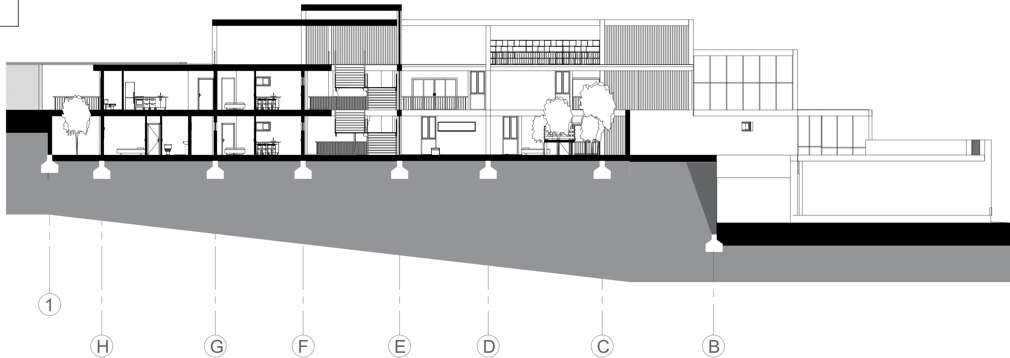
P-08 CORTE BB' ESC. 1:150
