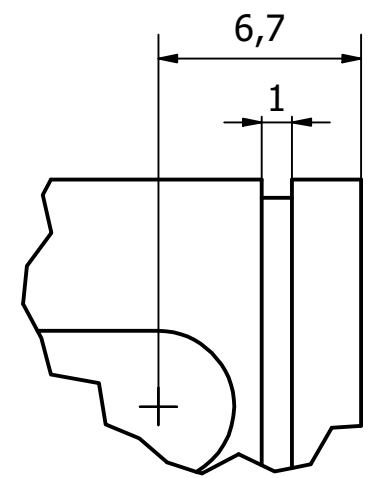
B ( 4 : 1 )
