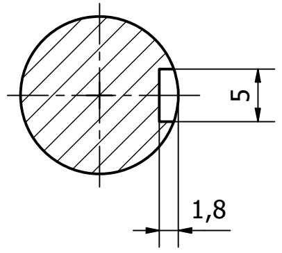
A-A ( 2 : 1 )
