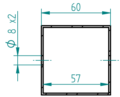
CORTE A-A
