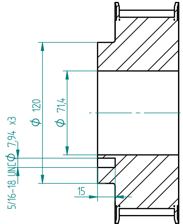
CORTE A-A
