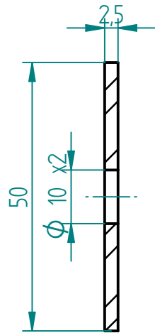
CORTE A-A
