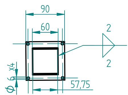
CORTE A-A
