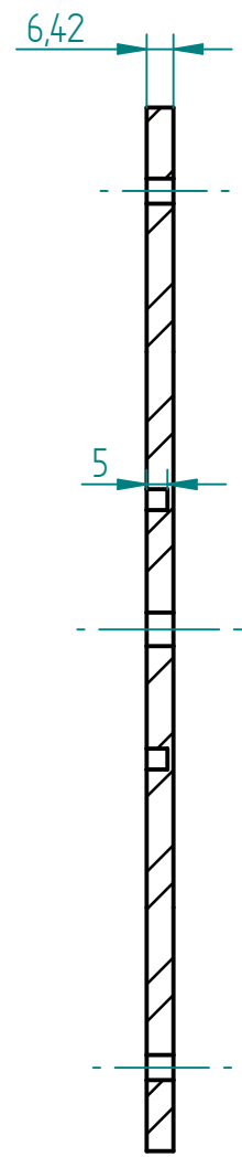
CORTE A-A
