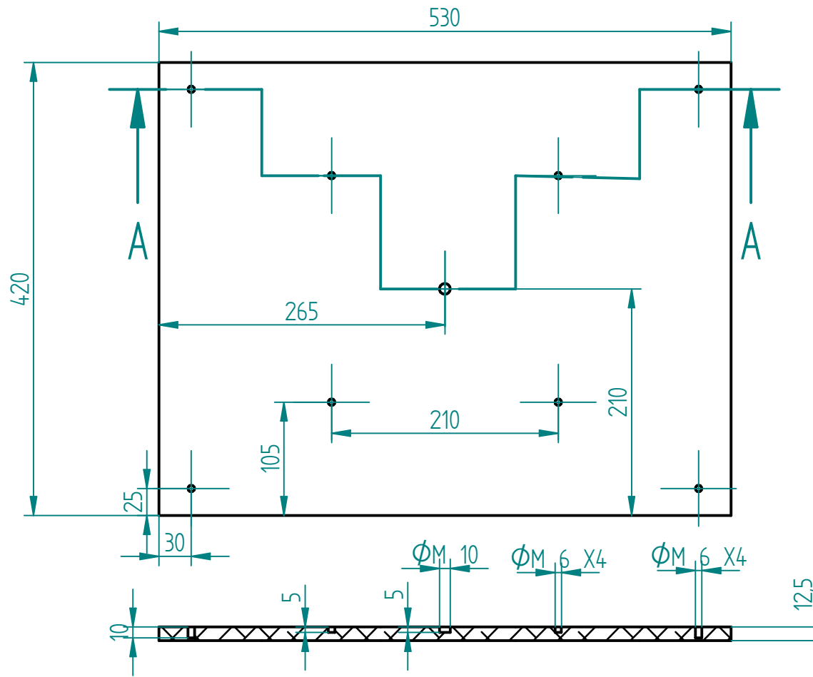
CORTE A-A
