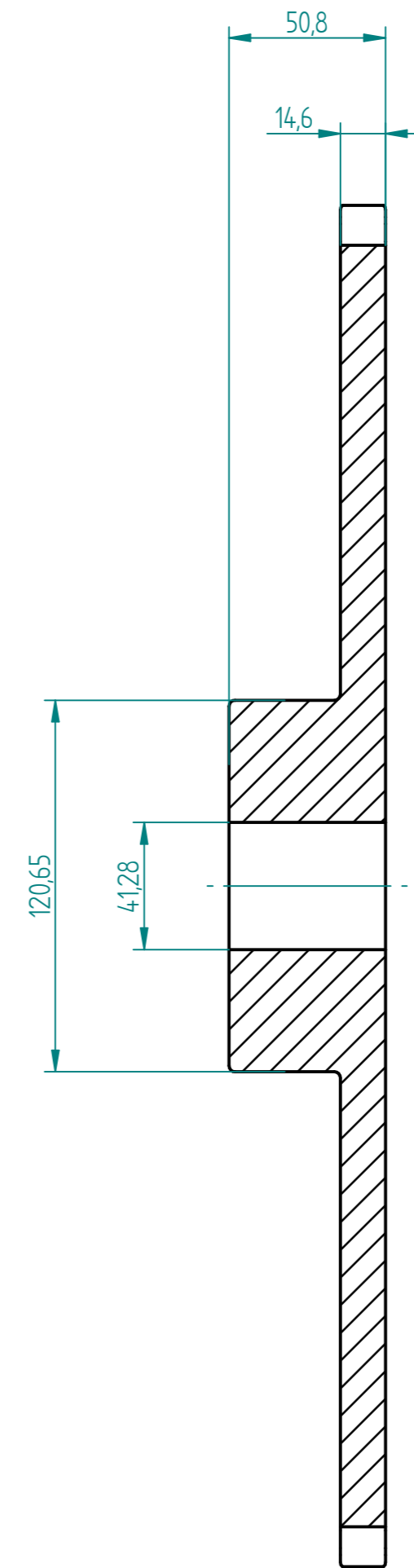
CORTE A-A
