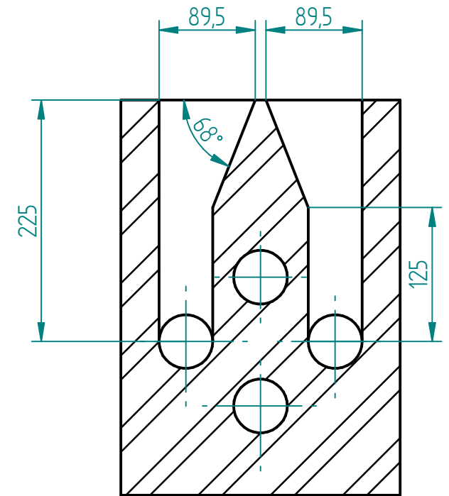
CORTE A-A
