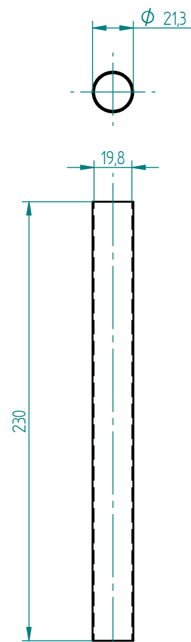
2. PERFIL CIRCULAR HUECO (ACOMODACIÓN)
