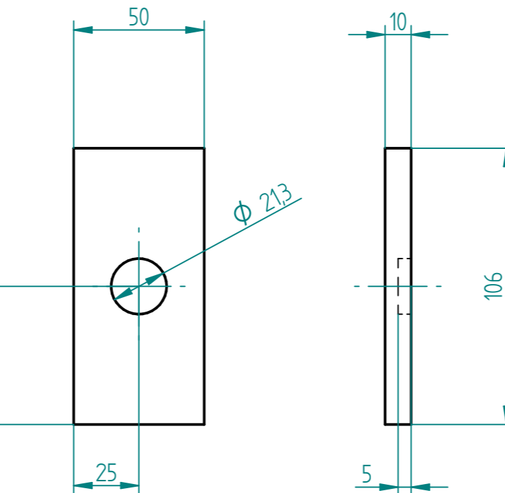
3. PLACA DE ACOMODAMIENTO
