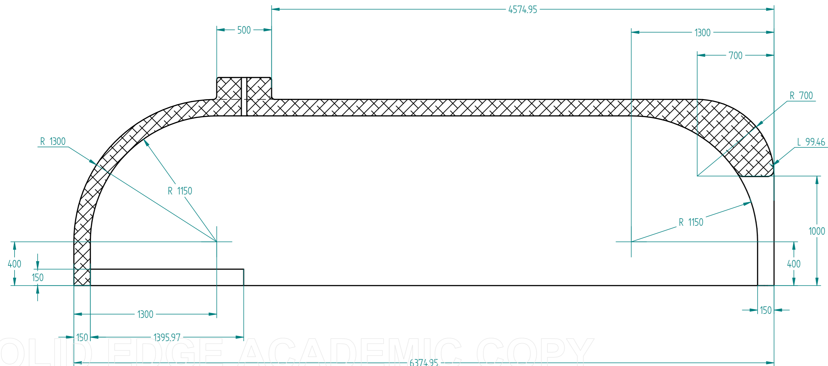
6374.95 CORTE A-A
