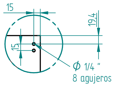
DETALLE B ESC: 1:5
