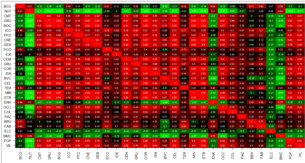
Matriz de correlación de las empresas listadas en bolsa
