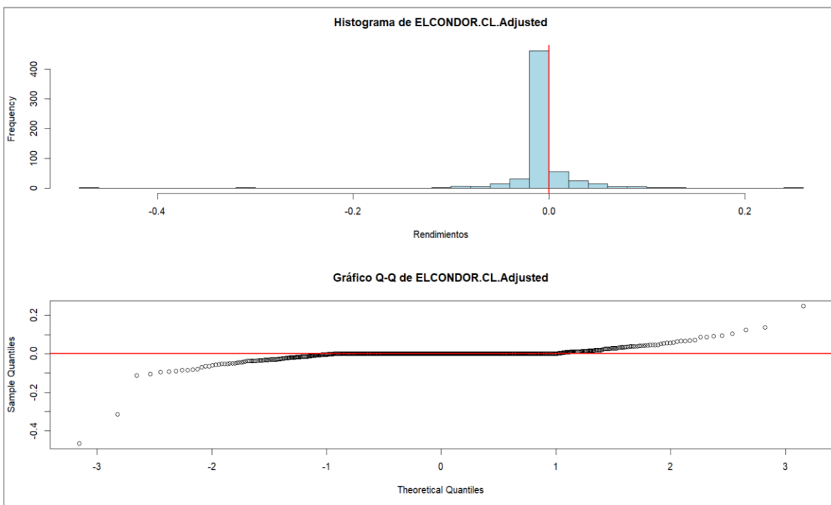
Histograma y gráfico Q-Q de los retornos de ELCONDOR.CL
