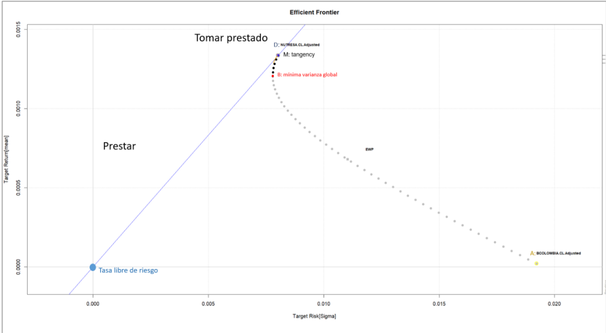
Frontera eficiente con el método MCD
