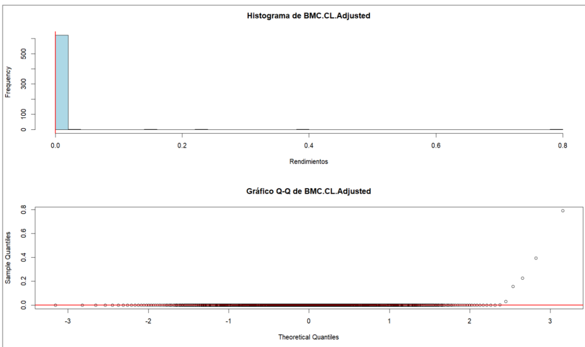
Histograma y gráfico Q-Q de los retornos de BMC.CL
