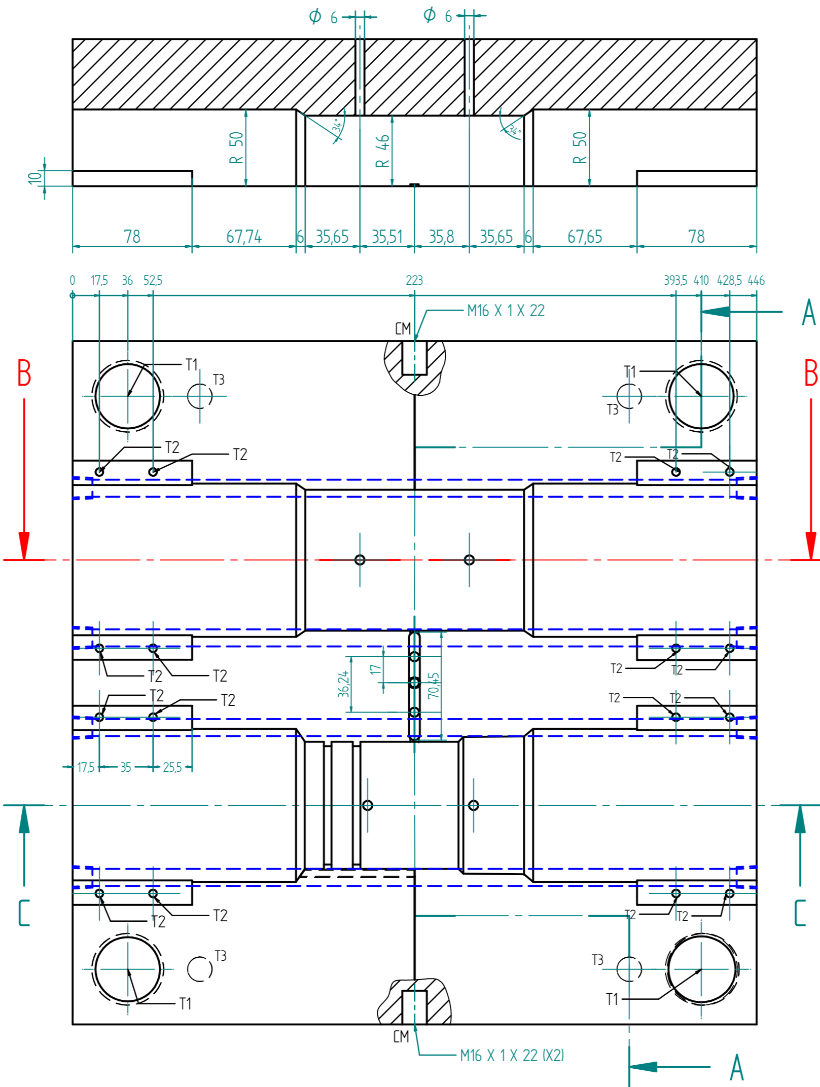
CORTE B-B
