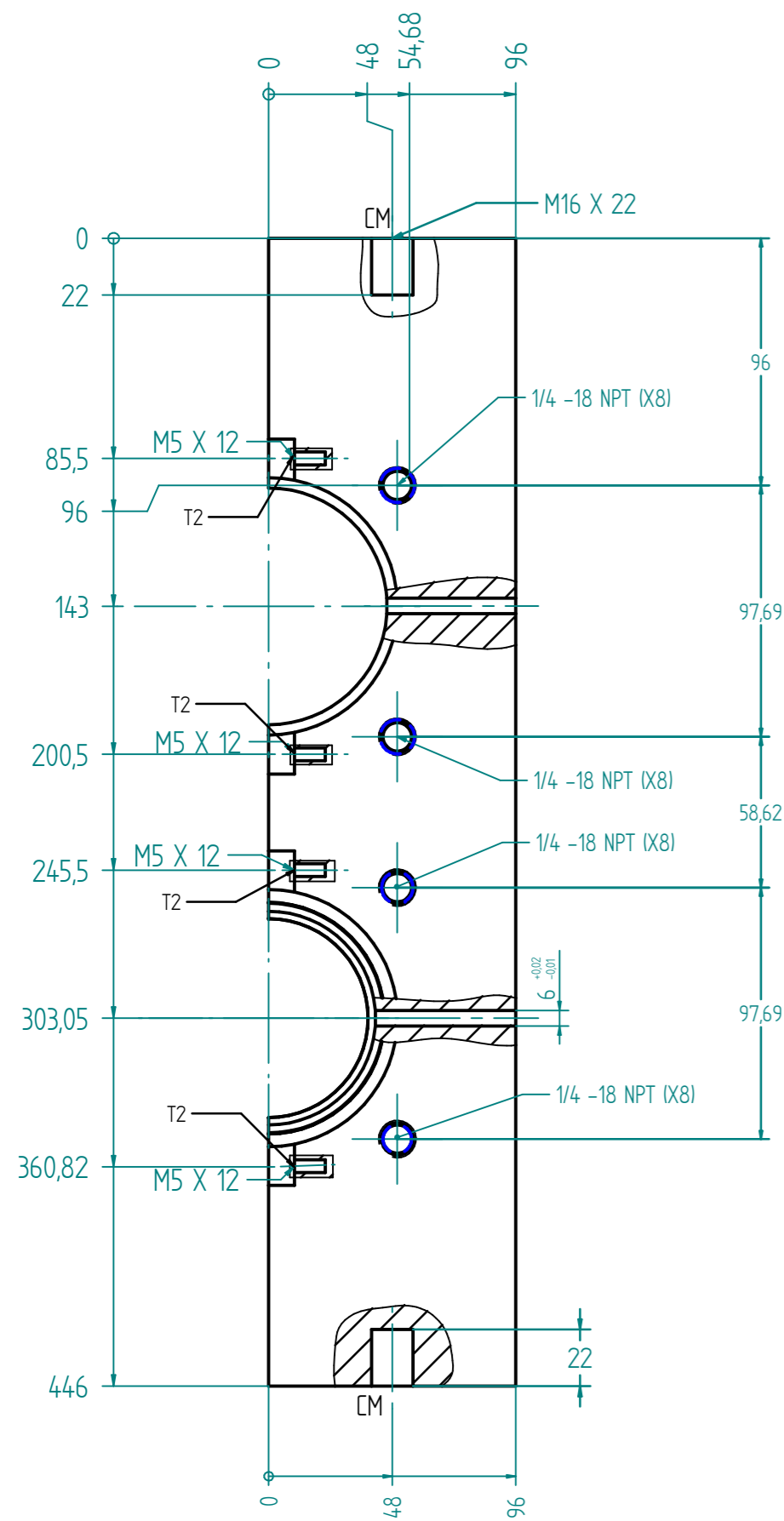
CORTE C-C
