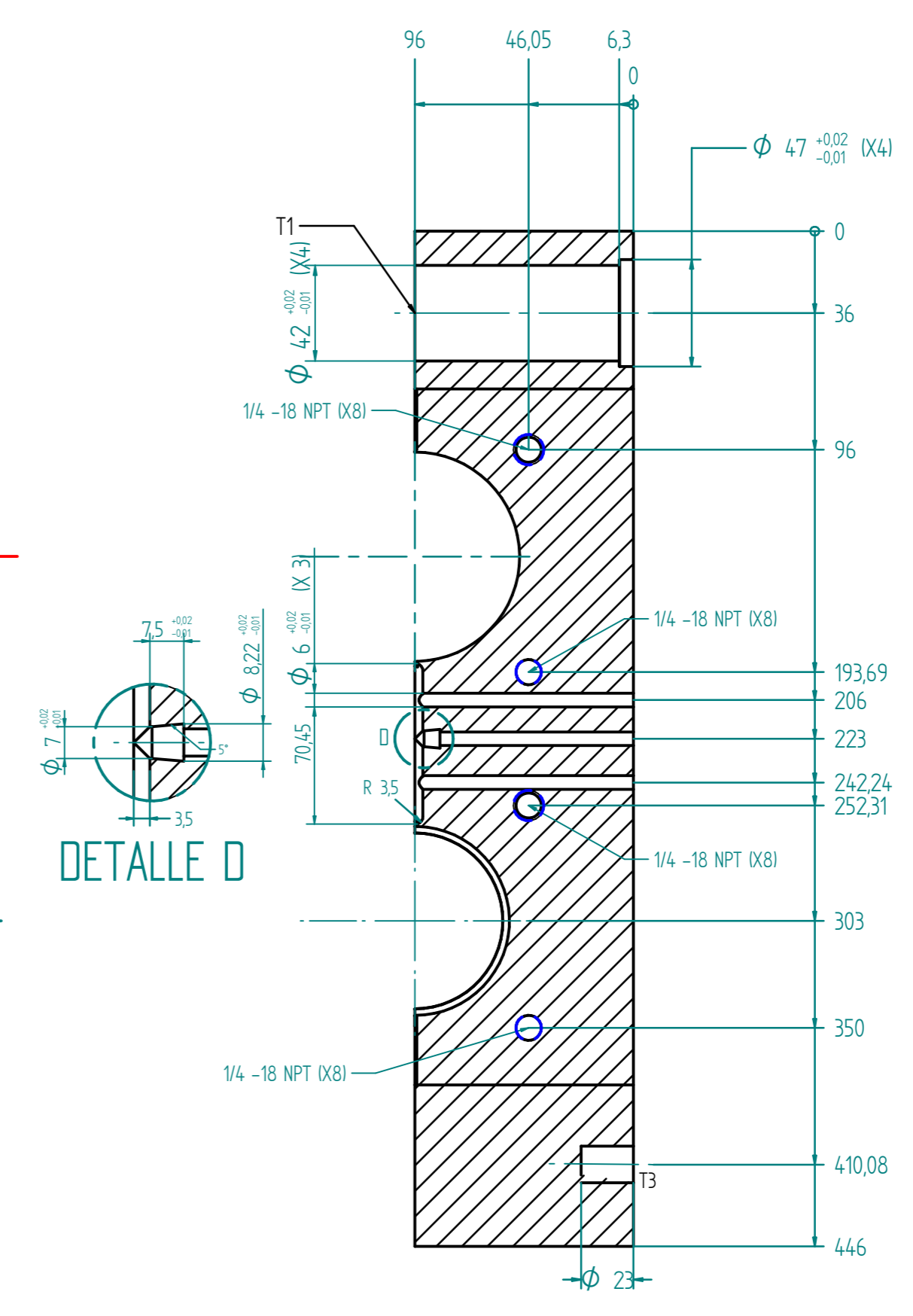
CORTE A-A
