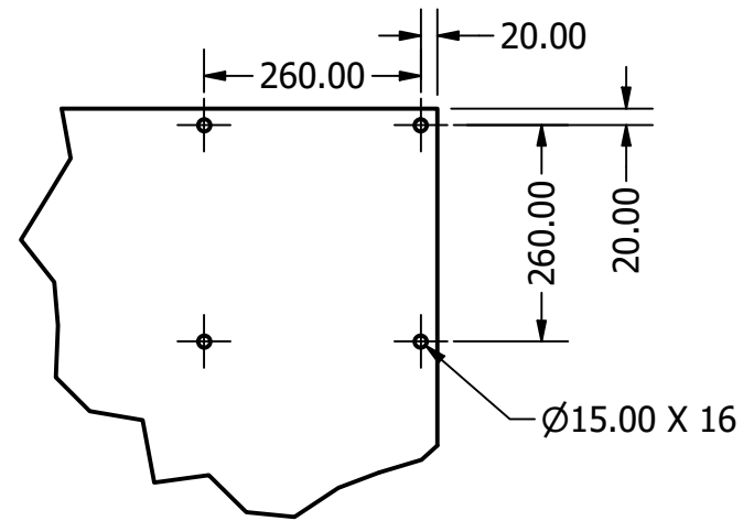
DETALLE A X 4 ESCALA 1 / 10
