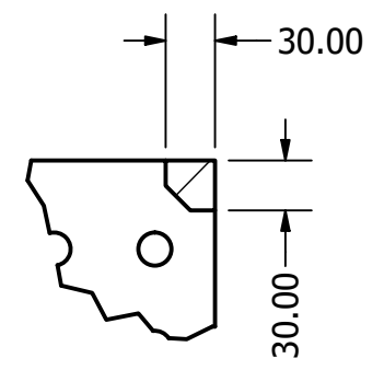
DETALLE E X 4 ESCALA 1 / 5
