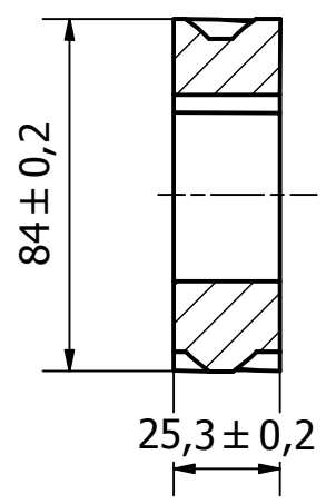
A-A ( 1 : 2 )
