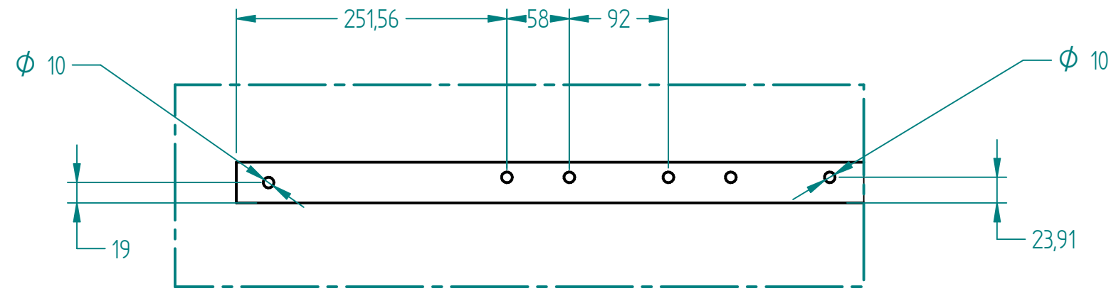
DETALLE A
