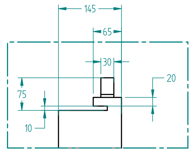
DETALLE B
