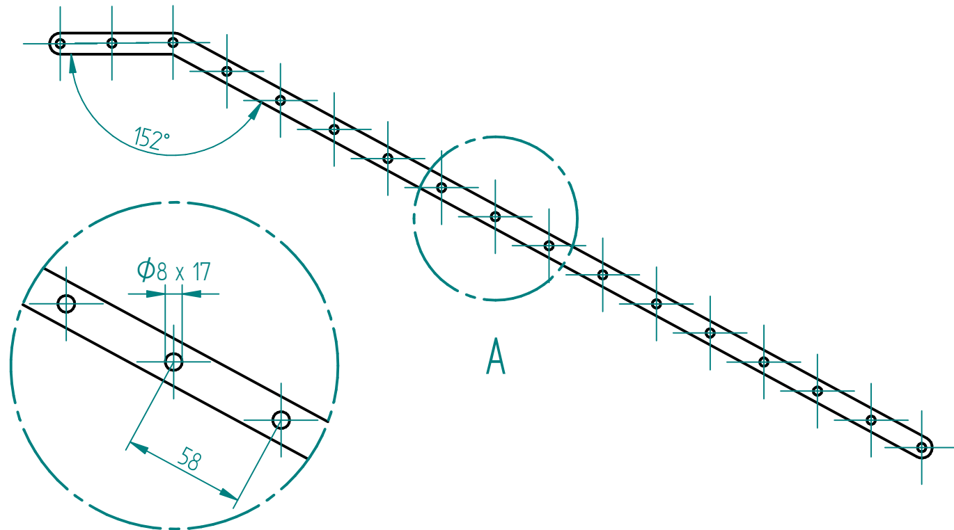
DETALLE A
