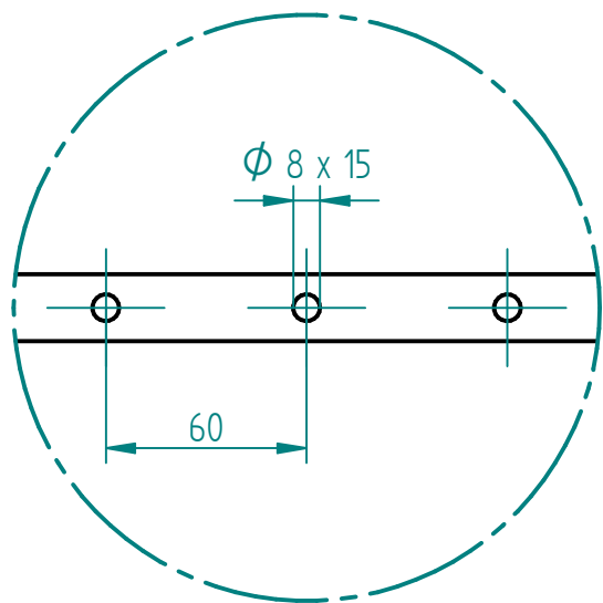
DETALLE A
