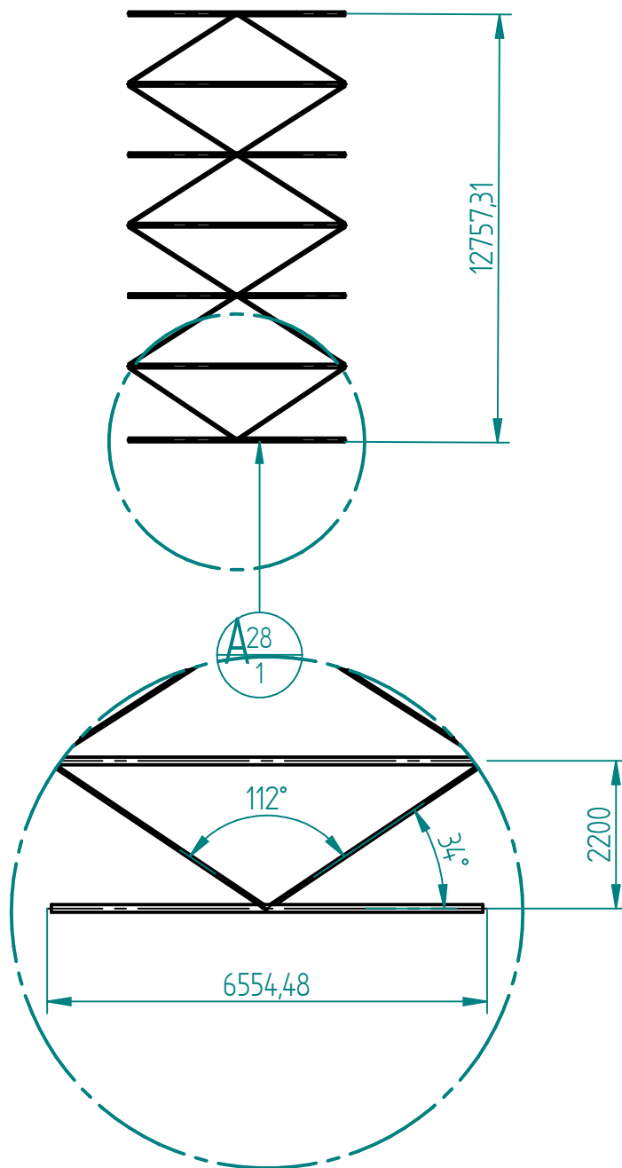
DETALLE A
