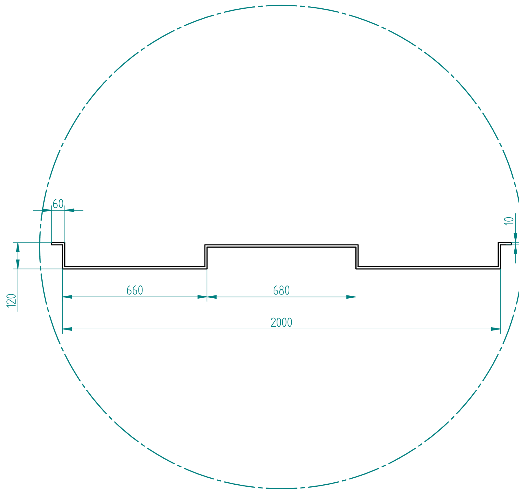
DETALLE A
