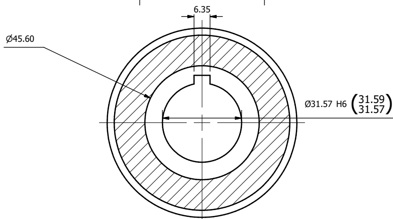
SECCIÓN K-K ESCALA 1:1
