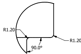
DETALLE M ESCALA 2 : 1
