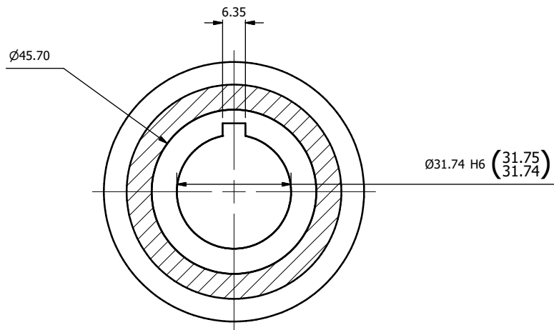
SECCIÓN K-K ESCALA 1 : 1
