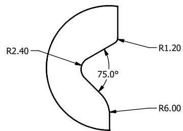
DETALLE N ESCALA 2 : 1
