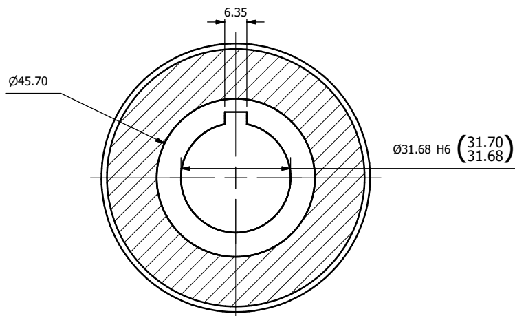
SECCIÓN K-K ESCALA 1 : 1
