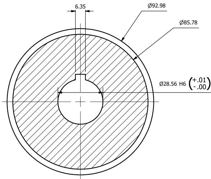
SECCIÓN N-N ESCALA 1 : 1
