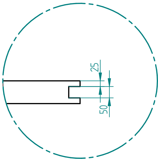
DETALLE F
